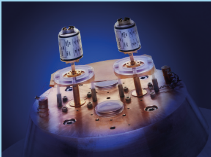
Калориметр для калибровки мощных высокочастотных термисторов
