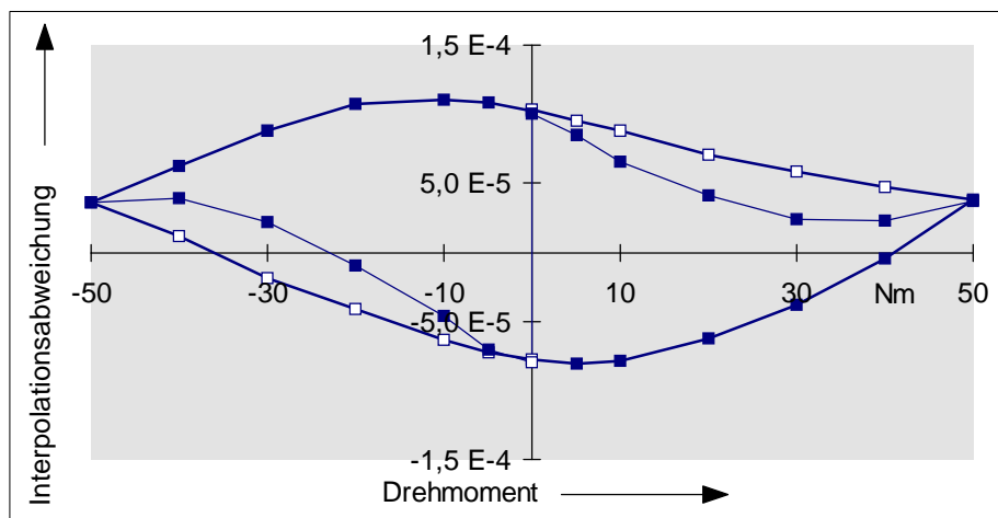
Bild 5b: Bereich der Regressionsabweichung (dicke Linien) für einen Wechseldrehmomentaufnehmer mit bekannter Vorgeschichte
