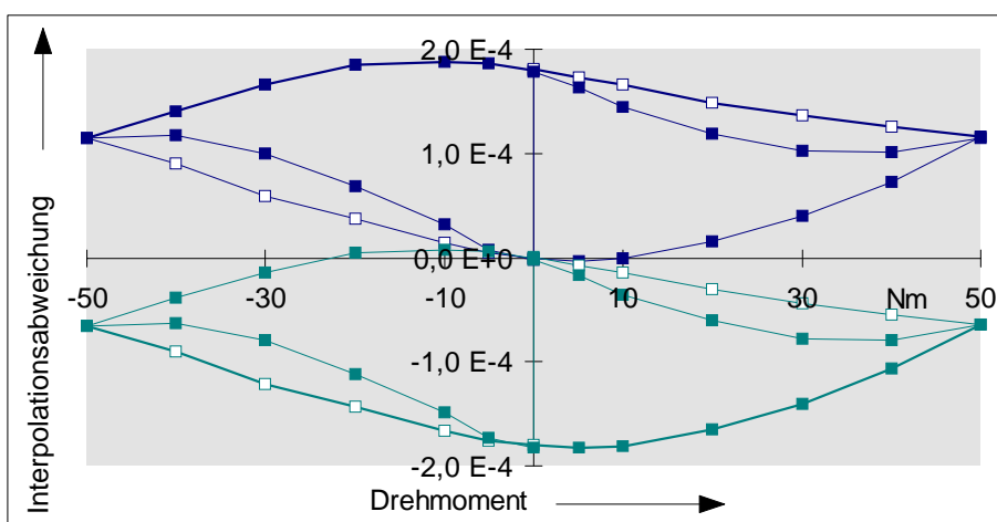
Bild 5a: Bereich der Regressionsabweichung (dicke Linien) für einen Wechseldrehmomentaufnehmer mit unbekannter Vorgeschichte
