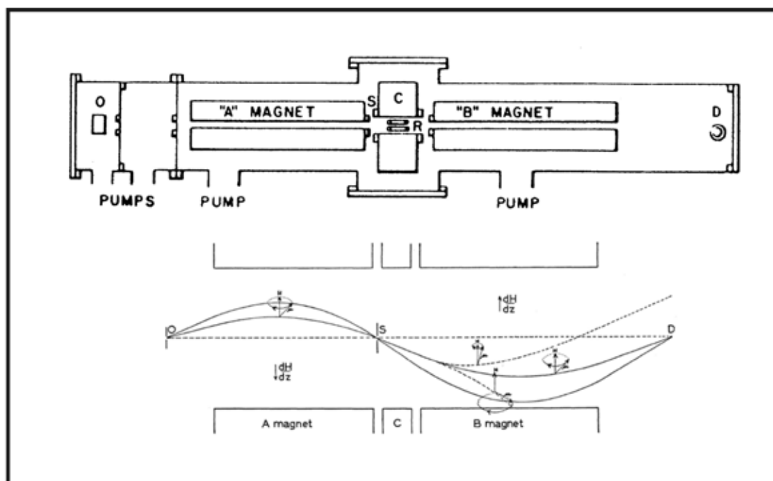
Bild 1: Skizze der Rabi-Apparatur aus den 1930er-Jahren (aus [2]) und Veranschaulichung der Atombahnen darunter (aus [4]), Erläuterungen im Text
