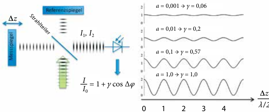
Bild 4: Erzeugung zweier zur Interferenz fähiger Lichtwellen mittels eines Interferometers (links). Im rechten Bereich ist die Intensität als Funktion der Verschiebung des Messspiegels für verschiedene Intensitätsverhältnisse ( a = I_1/I_2 ) dargestellt.
