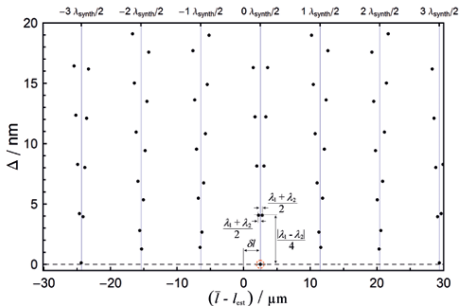
Bild 13: Typisches Koinzidenzmuster bei Verwendung von zwei Wellenlängen
